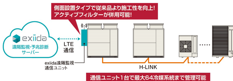
図 1: 「exiida 遠隔監視通信ユニット」接続時のシステム概要図(イメージ)
